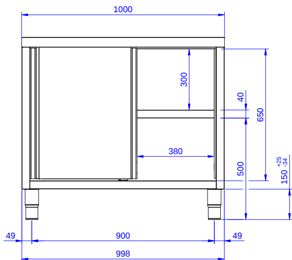
Fronte
